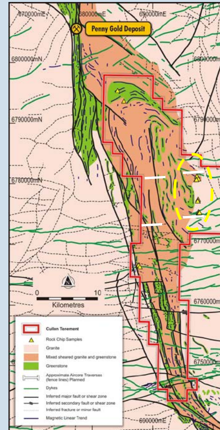
Bedrock Interpretation
